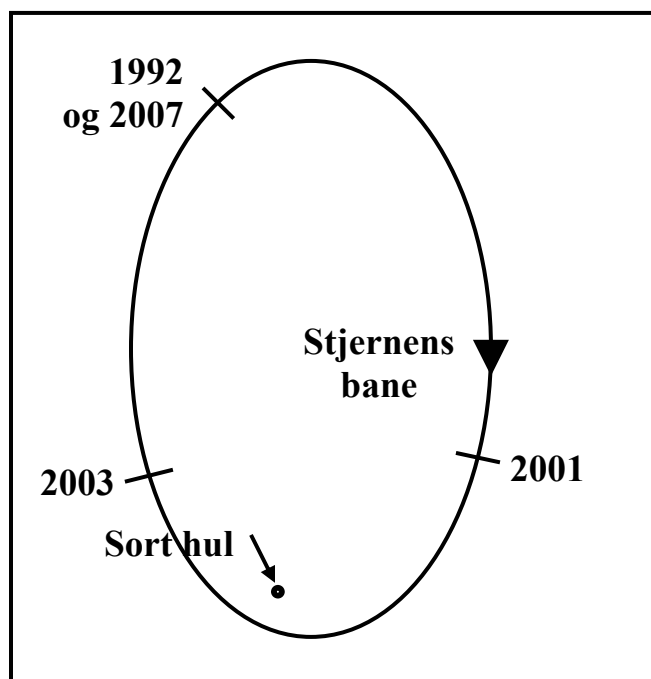
Figur 1. Det sorte hul i Mælkevejens centrum. Ellipsen viser den bane, som vores stjerne, S2, har fulgt i et enkelt omløb på 15 år siden 1992.
